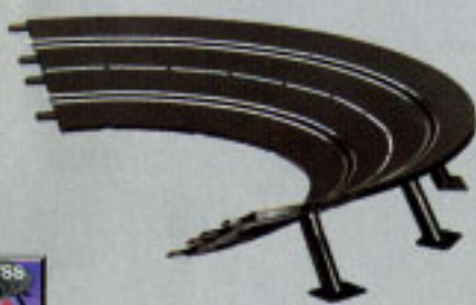
20574 Steilkurve 1/30° ohne Außenrandstreifen 6 Stück = 180° Pgröße: ca. 36,5 x 21,5 x 10 cm Gewicht: ca. 750 g Bestelleinheit: 1
