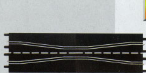
20516 Engstelle Pgröße: ca. 39,6 x 20,5 x 2 cm Gewicht: ca. 490 g Bestelleinheit: 1
