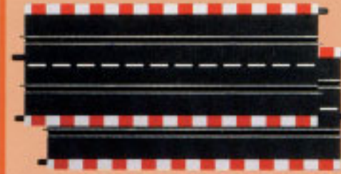
71509 Doppelgerade 2 Stück a 43 cm Pg.: ca. 48 x 18,3 x 2,5 cm Gewicht: ca. 500 g Bestelleinheit: 4
