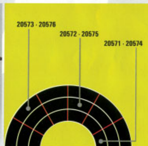
20573 Kurve 3/30° ohne Außenrandstreifen 6 Stück für 6-spurigen Ausbau = 180° Pgröße: ca. 47,3 x 22,5 x 5,6 cm Gewicht: ca. 1570 g Bestelleinheit: 1
