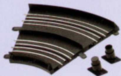
77524 Steilkurve aus 4 Elementen mit 17° Neigungswinkel - Inhalt: 4 Steilkurven, 8 Stützen, Bahnstückverriegelungen Packungsgröße: ca. 35,8 x 18,7 x 6,7 cm Gewicht: ca. 395 g Bestelleinheit: 2
