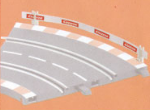
72556 Leitplanken-Set Gewicht: ca. 150 g Pgröße: ca. 10 x 10 x 0,3 cm Bestelleinheit: 4
